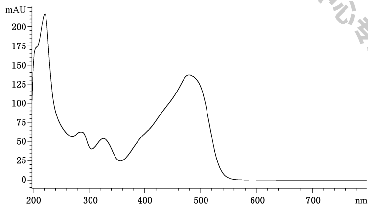
图 B.5 颜料橙 5 标准品的紫外可见吸收光谱图
