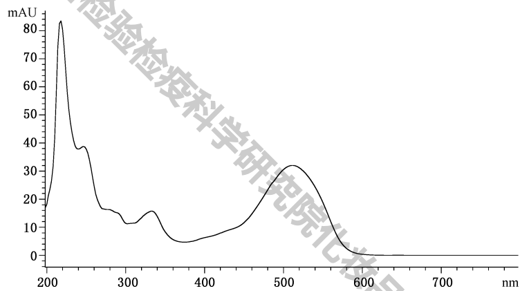
图 B.4 颜料红 53：1 标准品的紫外可见吸收光谱图
