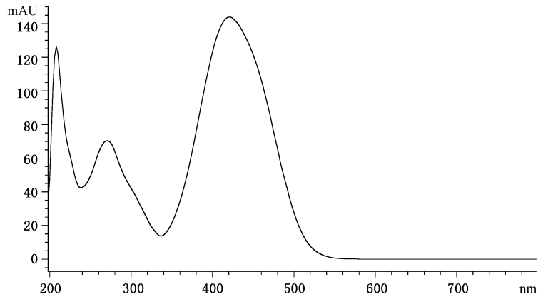
图 B.3 酸性黄 36 标准品的紫外可见吸收光谱图
