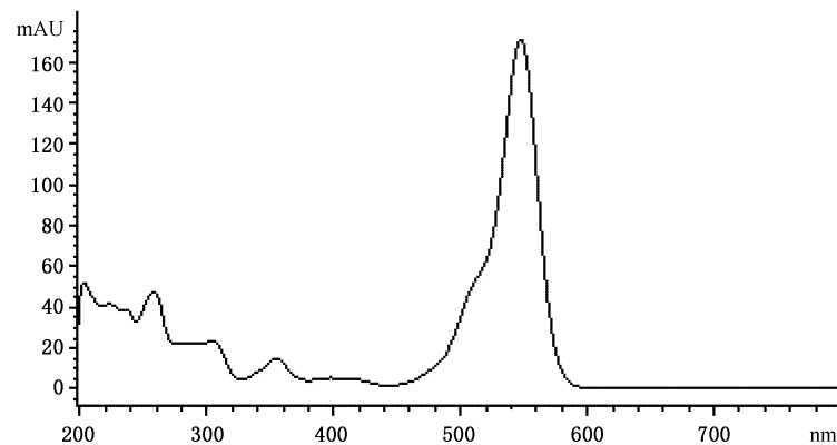
图 B.2 罗丹明 B 标准品的紫外可见吸收光谱图
