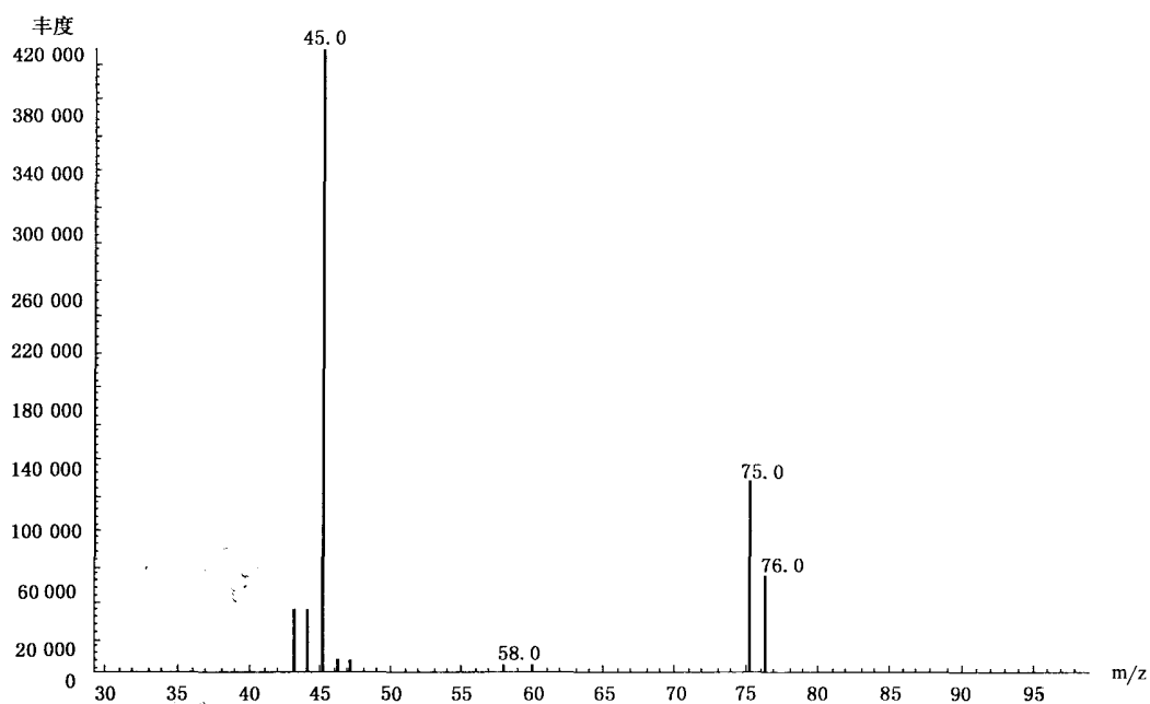
图 B.2 二甘醇的质谱图
