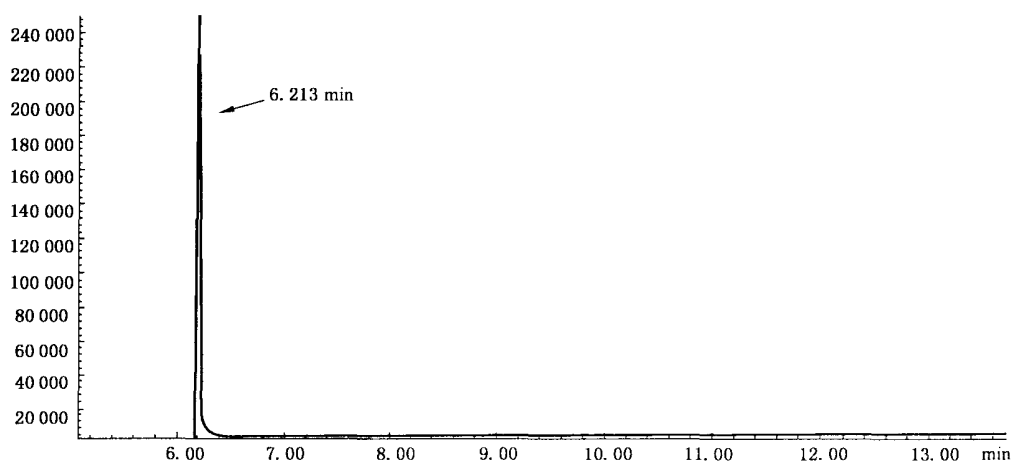
图 B.1 二甘醇的总离子流色谱图
